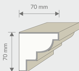
model: 165
